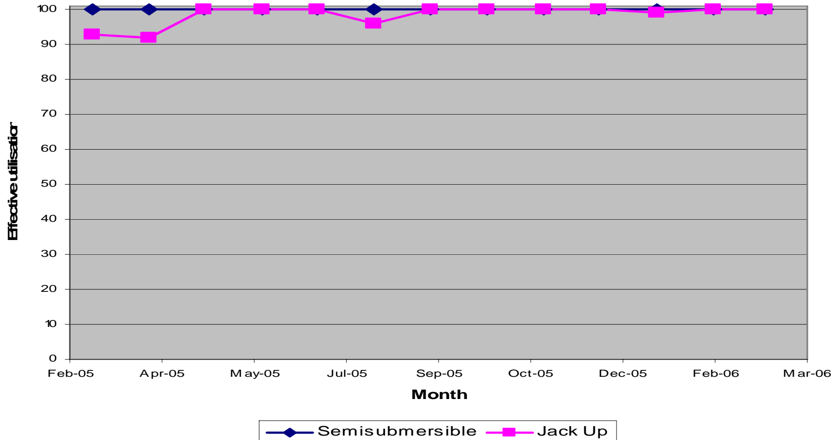
North Sea Effective Rig Utilisation
