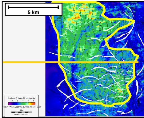
Upper F3 sand: Maximum Amplitude
