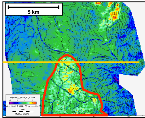
Middle F3 sand: Maximum Amplitude
